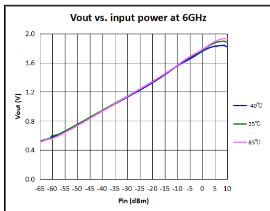
图 11 6000MHz 全温检波曲线
