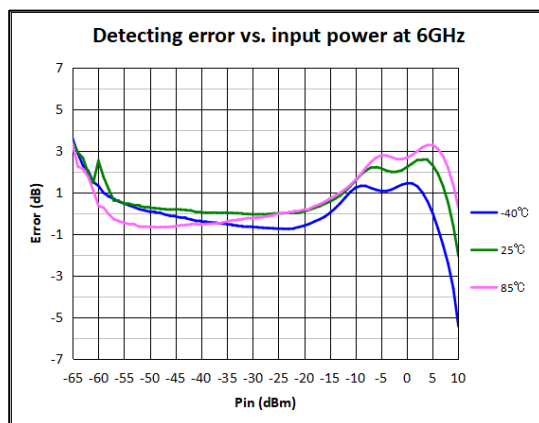
图 12 6000MHz 全温检波对数误差
