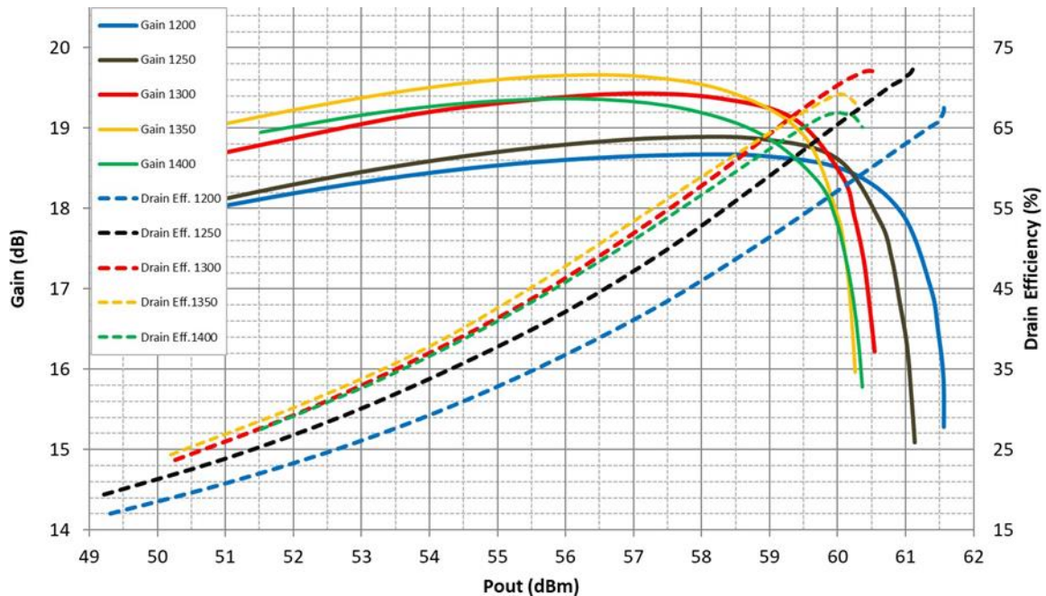
增益、漏极效率与输出功率的性能曲线图
